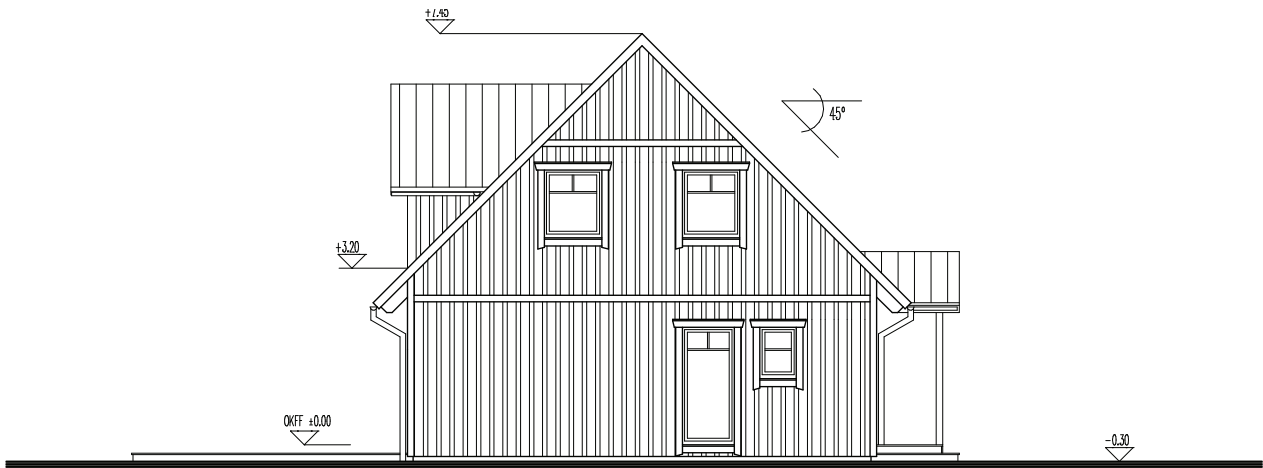
Süd – Westansicht
