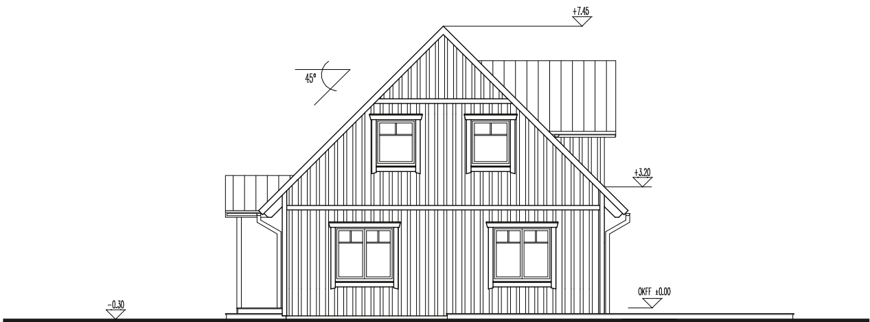
Nord – Ostansicht
